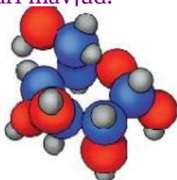
Glyukoza molekulasi
