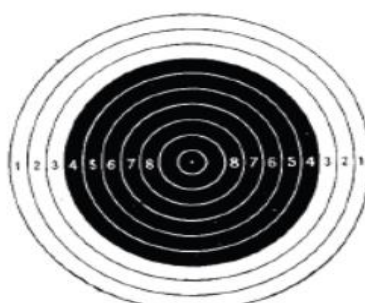
2-rasm. 8 raqamli nishon. Qora doiraning diametri – 31 mm. O'nlikning diametri – 1 mm
