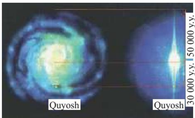
102-rasm. Galaktikamizning ust va yon tomondan ko‘rinishi.
