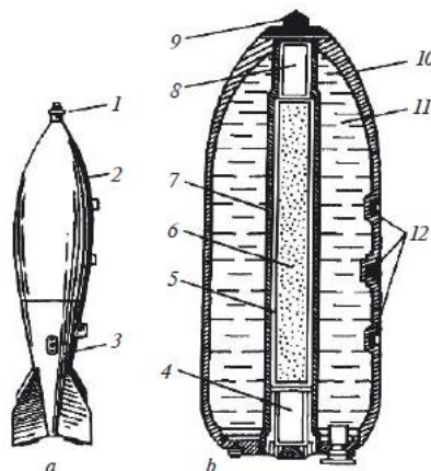
4-rasm. 340 kilogramm og‘irlidagi MS-1 rusumli kimyoviy bomba: a — umumiy ko‘rinishi; b — kesilgan holda ko‘rinishi; 1, 9 — bosh portlagich moslama; 2, 10 — korpus; 3 — stabilizator; 4—8 — vtulkalar; 5 — gofirlangan kartondan tayyorlangan silindr; 6 — portlovchi zaryad; 7 — portlovchi zaryadni solish uchun mo‘ljallangan stakan; 11 — zaharlovchi modda; 12 — bombani osib qo‘yish uchun mo‘ljallangan ilgaklar.
